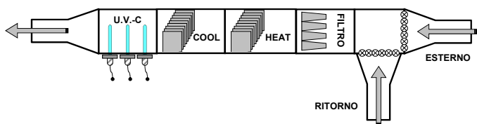
CENTRALE TRATTAMENTO ARIA CON CANALIZZAZIONE
